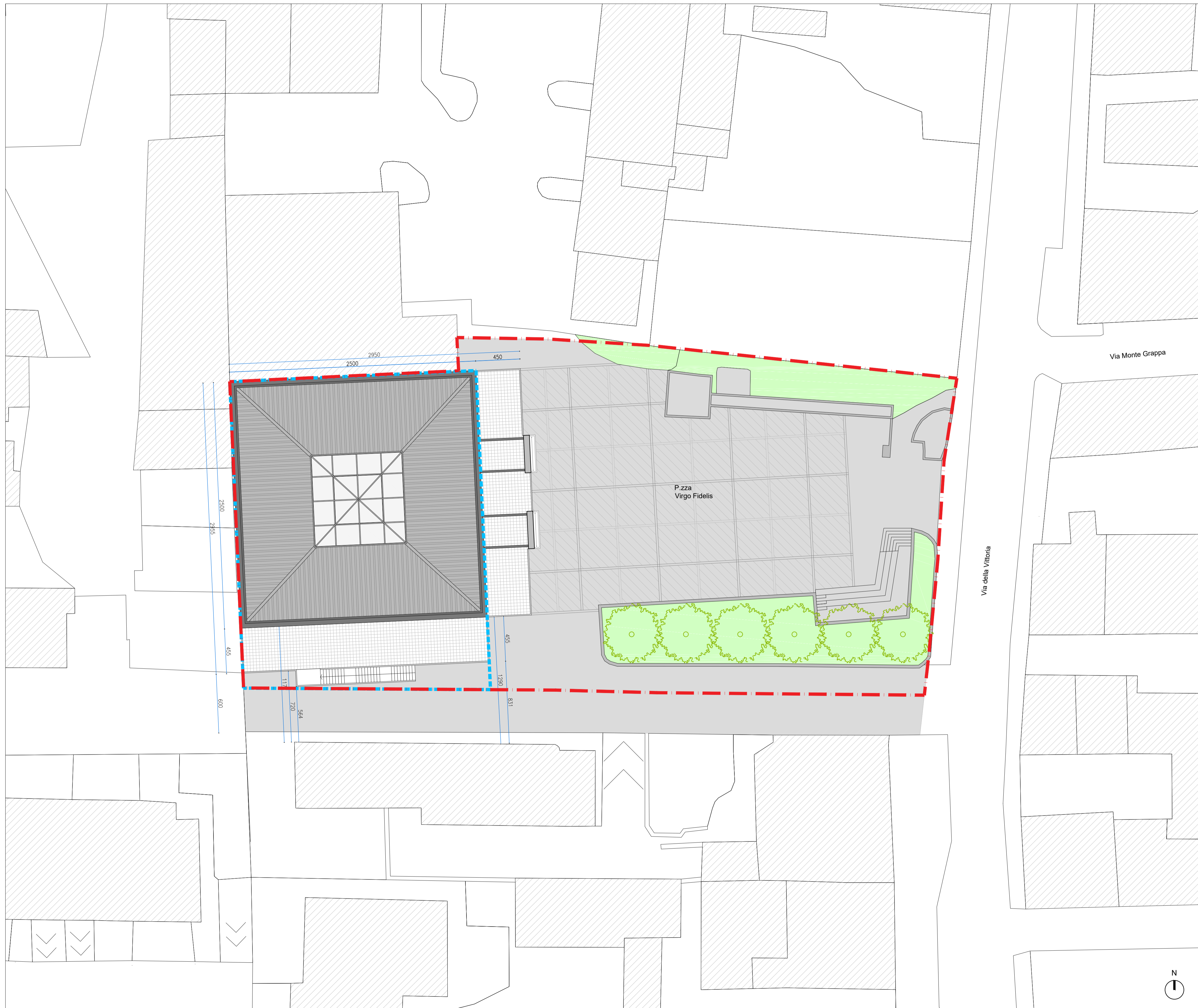
PLANIMETRIA GENERALE DELL'AREA DI INTERVENTO - SCALA 1:200
