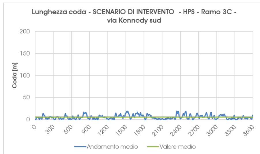
Grafico 39 – Scenario di Intervento – Accodamento medio – ramo 3C – Ora di punta della sera
