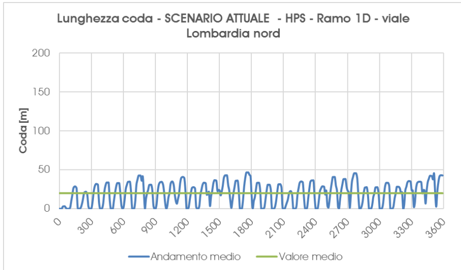
Grafico 20 – Scenario Attuale – Accodamento medio – ramo 1D – Ora di punta della sera
