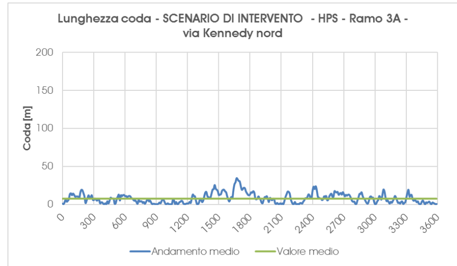
Grafico 35 – Scenario di Intervento – Accodamento medio – ramo 3A – Ora di punta della sera
