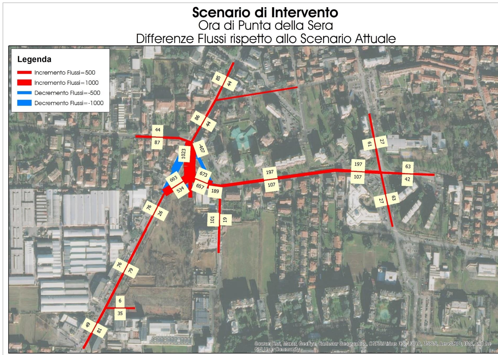
Figura 51 – Scenario di Intervento – Ora di punta della sera – Differenze Flussi rispetto allo Scenario Attuale
