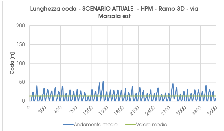
Grafico 31 – Scenario Attuale – Accodamento medio – ramo 3D – Ora di punta della mattina
