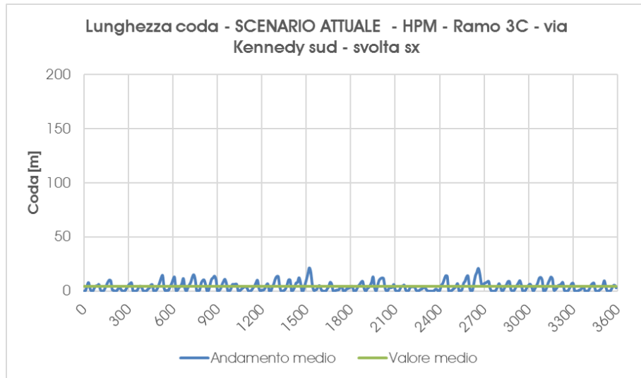
Grafico 30 – Scenario Attuale – Accodamento medio – ramo 3C – svolta SX – Ora di punta della mattina
