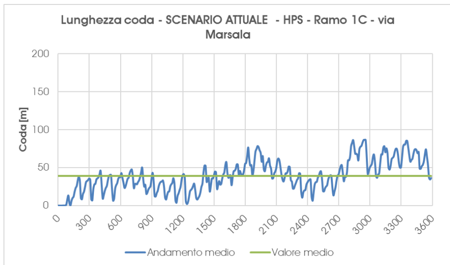
Grafico 19 – Scenario Attuale – Accodamento medio – ramo 1C – Ora di punta della sera
