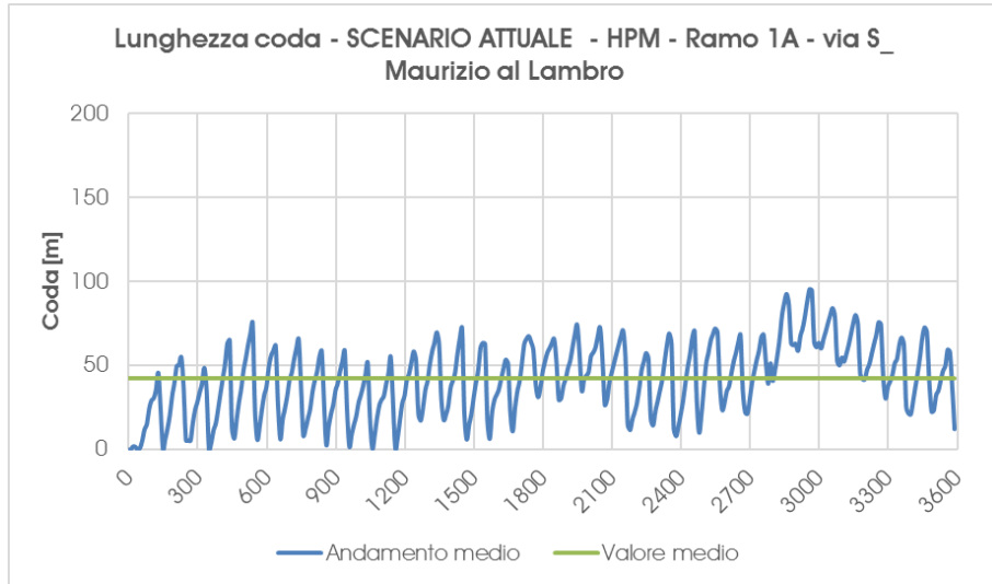
Grafico 7 – Scenario Attuale – Accodamento medio – ramo 1A – Ora di punta della mattina
