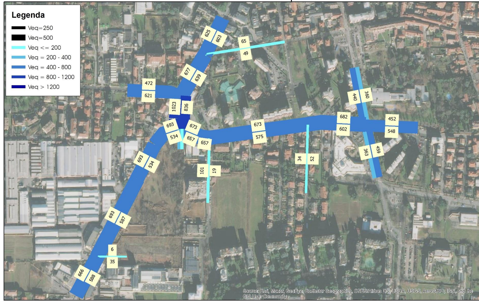
Figura 47 – Scenario di Intervento – Ora di punta della sera – Flussogramma
