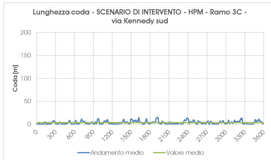
Grafico 29 – Scenario di Intervento – Accodamento medio – ramo 3C – Ora di punta della mattina
