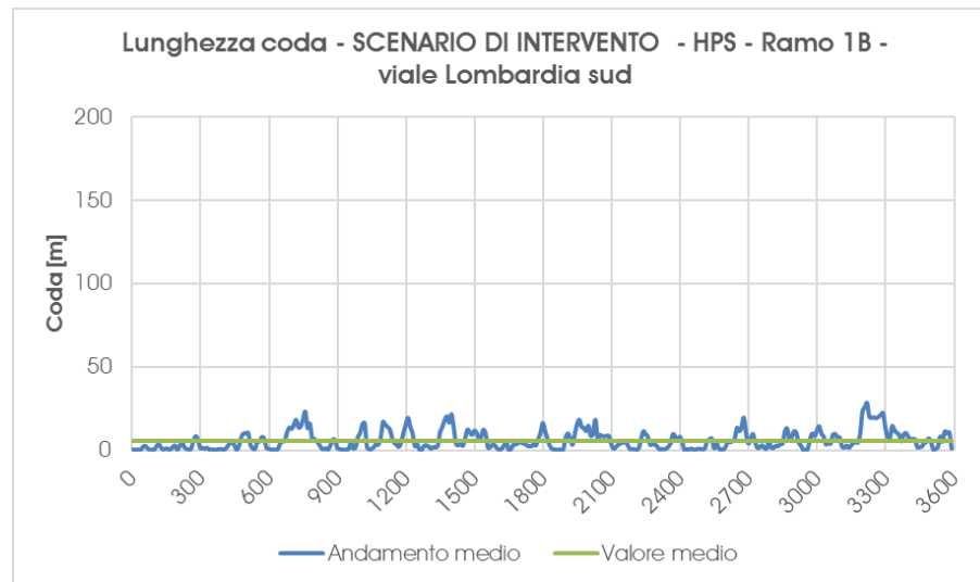
Grafico 18 – Scenario di Intervento – Accodamento medio – ramo 1B – Ora di punta della sera
