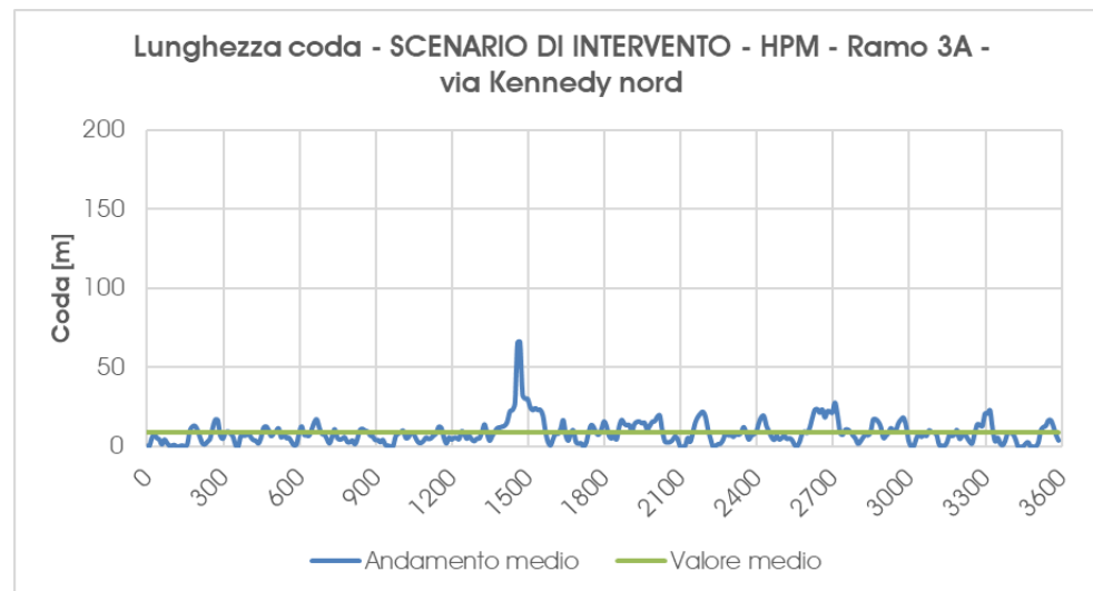
Grafico 25 – Scenario di Intervento – Accodamento medio – ramo 3A – Ora di punta della mattina
