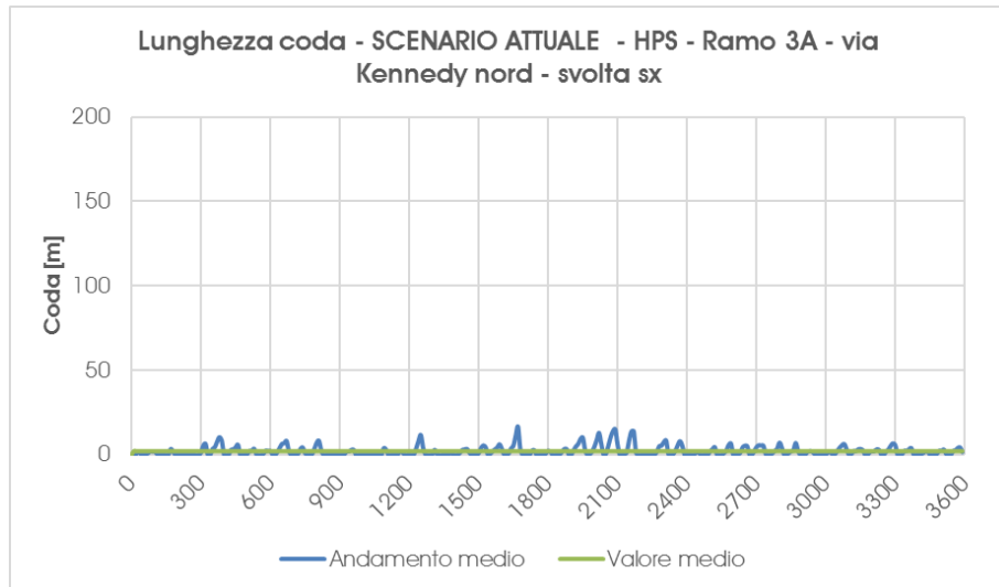
Grafico 34 – Scenario Attuale – Accodamento medio – ramo 3A svolta SX– Ora di punta della sera
