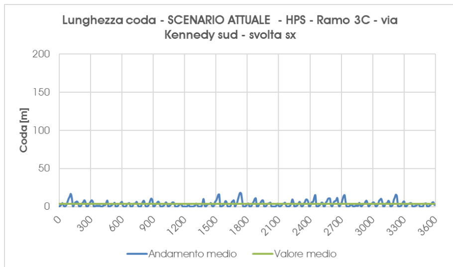
Grafico 40 – Scenario Attuale – Accodamento medio – ramo 3C – svolta SX – Ora di punta della sera
