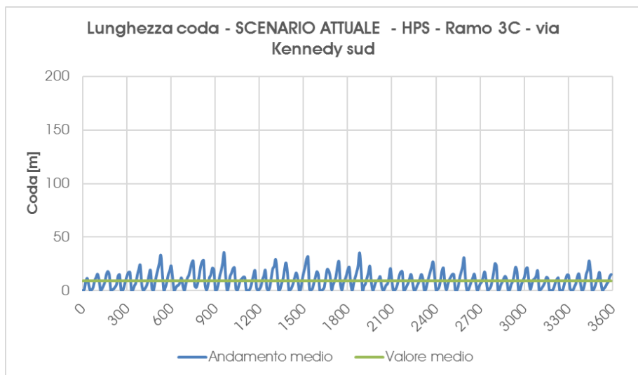
Grafico 37 – Scenario Attuale – Accodamento medio – ramo 3C – Ora di punta della sera
