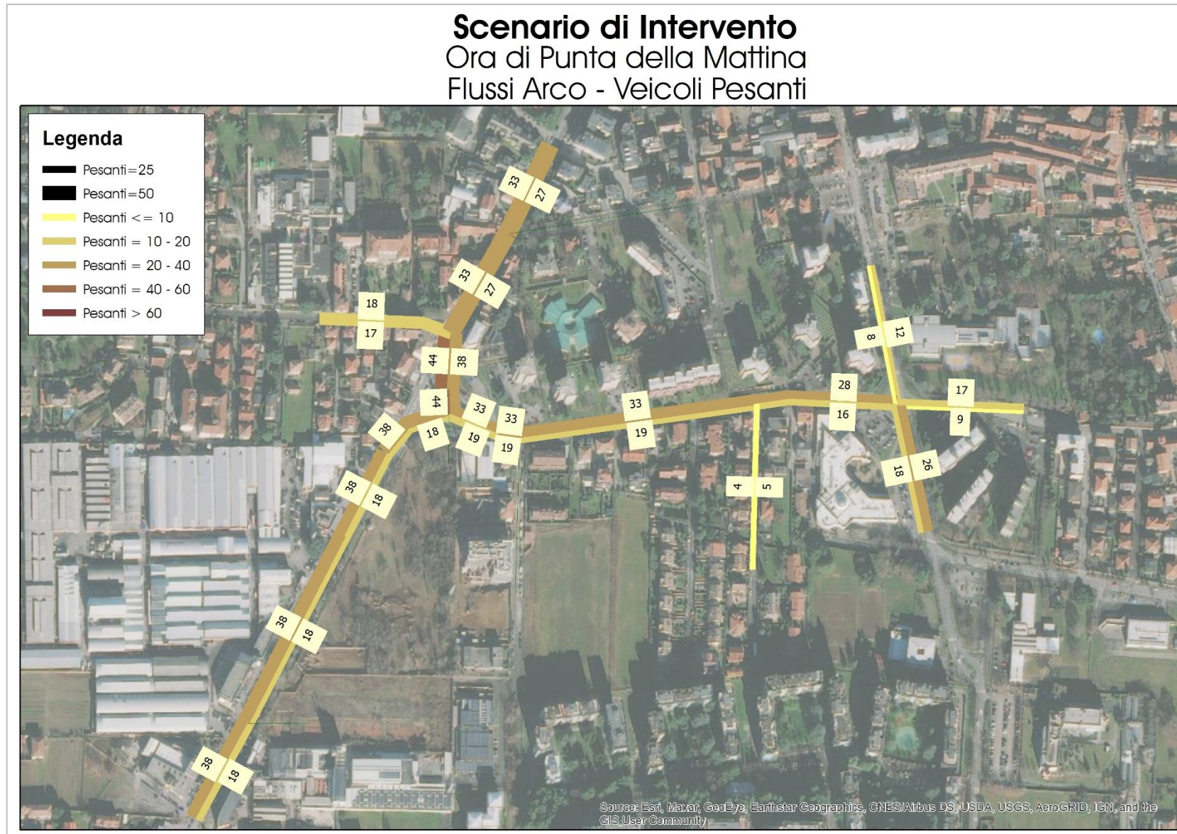
Figura 44 – Scenario di Intervento – Ora di punta della mattina – Flussogramma – Veicoli Pesanti
