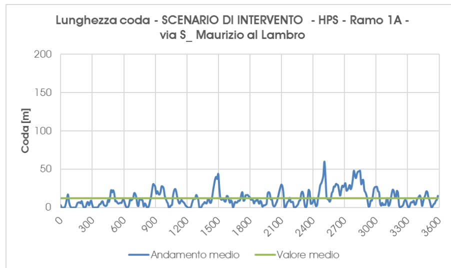
Grafico 17 – Scenario di Intervento – Accodamento medio – ramo 1A – Ora di punta della sera
