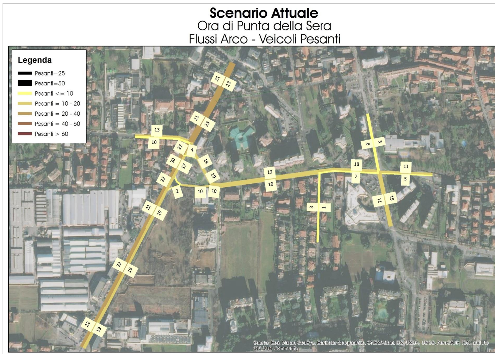
Figura 34 – Scenario Attuale – Ora di punta della sera – Flussogramma – Veicoli Pesanti
