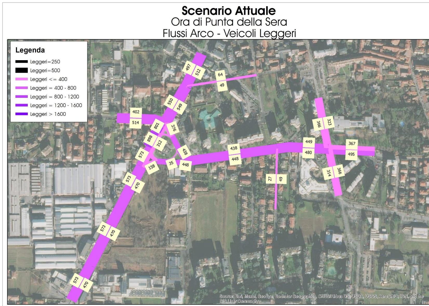
Figura 33 – Scenario Attuale – Ora di punta della sera – Flussogramma – Veicoli Leggeri
