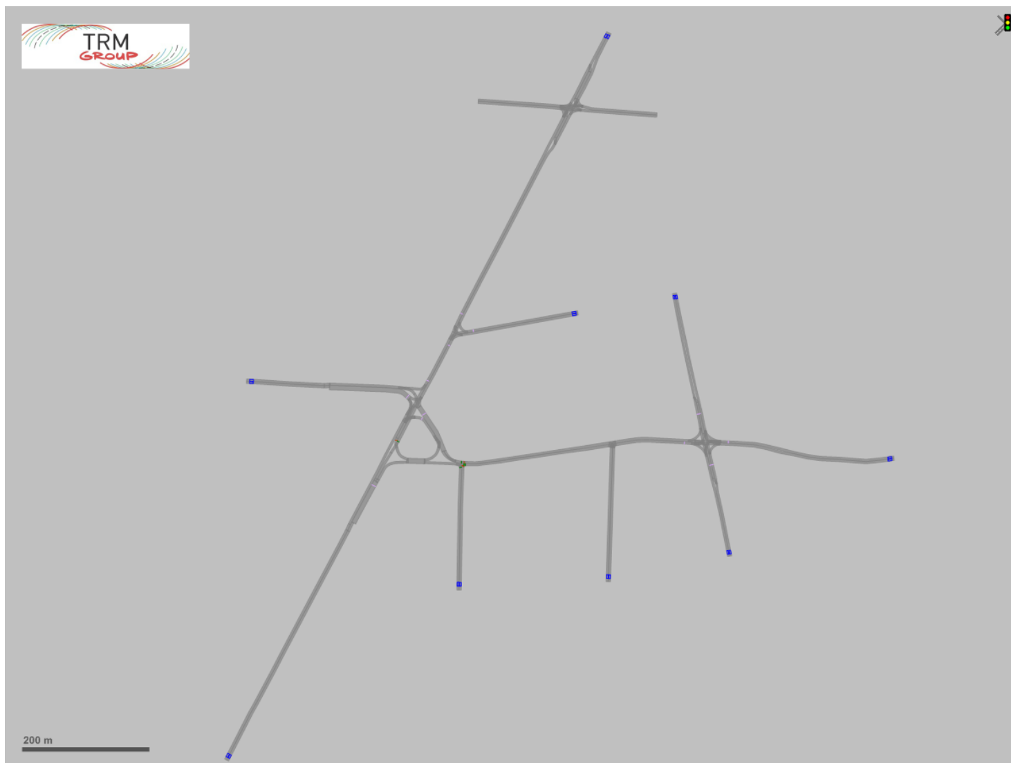
Figura 57 – Scenario Attuale – Rete modellizzata con il software VISSIM
