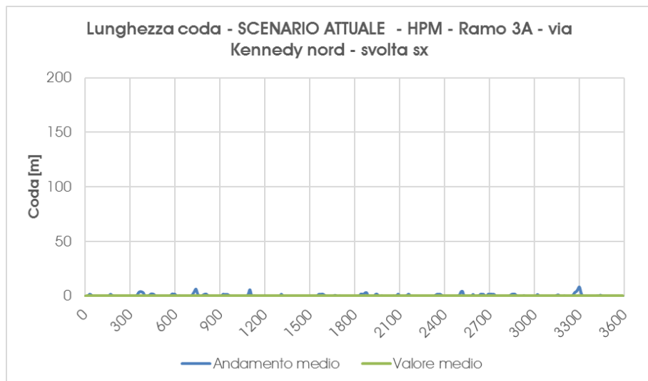
Grafico 24 – Scenario Attuale – Accodamento medio – ramo 3A svolta SX– Ora di punta della mattina
