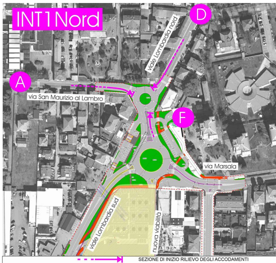
Figura 62 – Scenario di intervento – Intersezione 1 Nord
