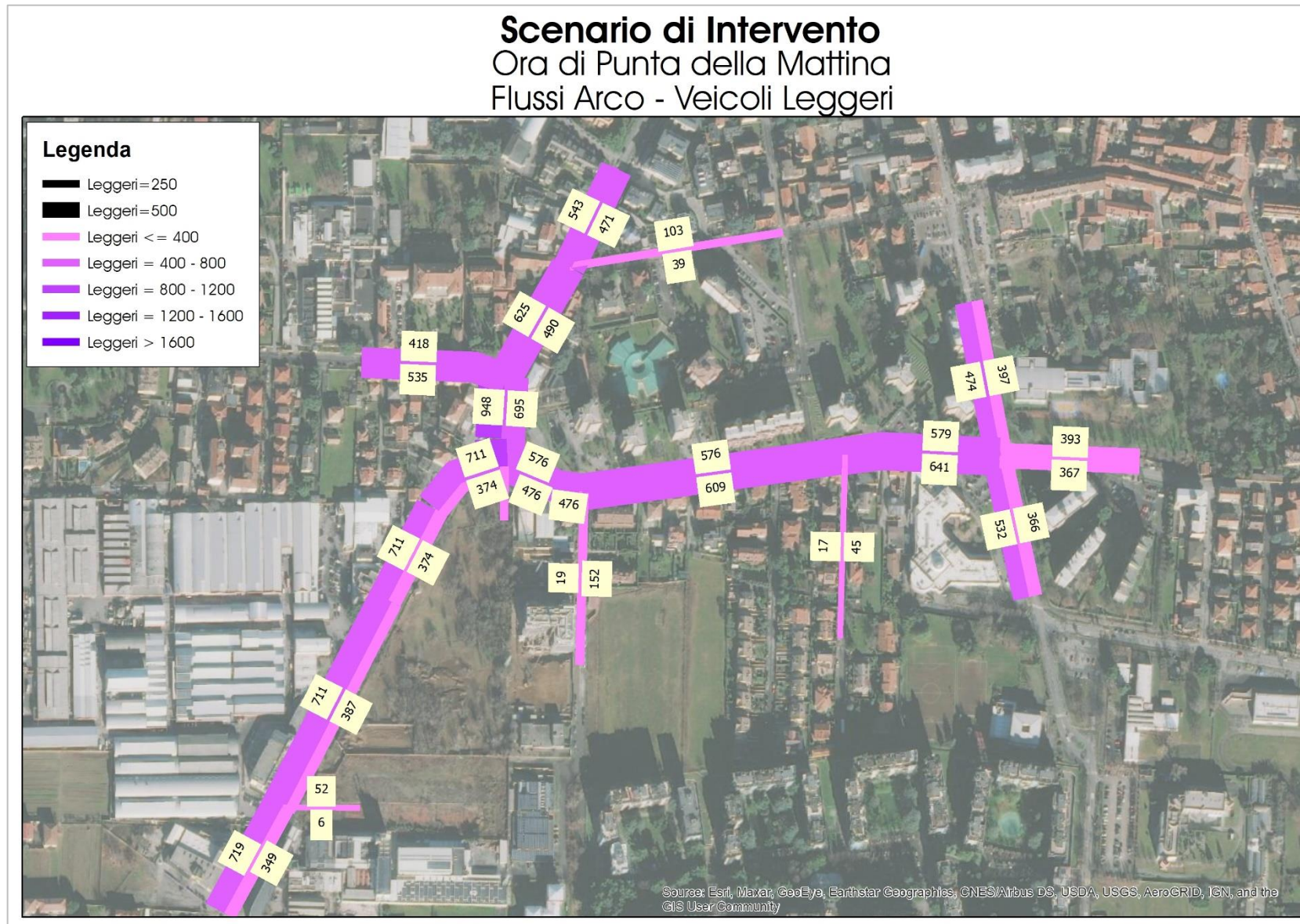
Figura 43 – Scenario di Intervento – Ora di punta della mattina – Flussogramma – Veicoli Leggeri
