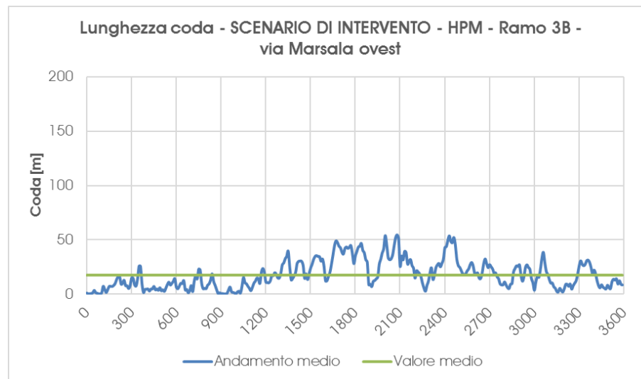
Grafico 28 – Scenario di Intervento – Accodamento medio – ramo 3B – Ora di punta della mattina
