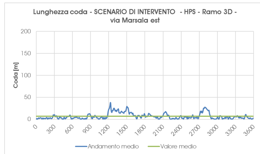
Grafico 42 – Scenario di Intervento – Accodamento medio – ramo 3D – Ora di punta della sera
