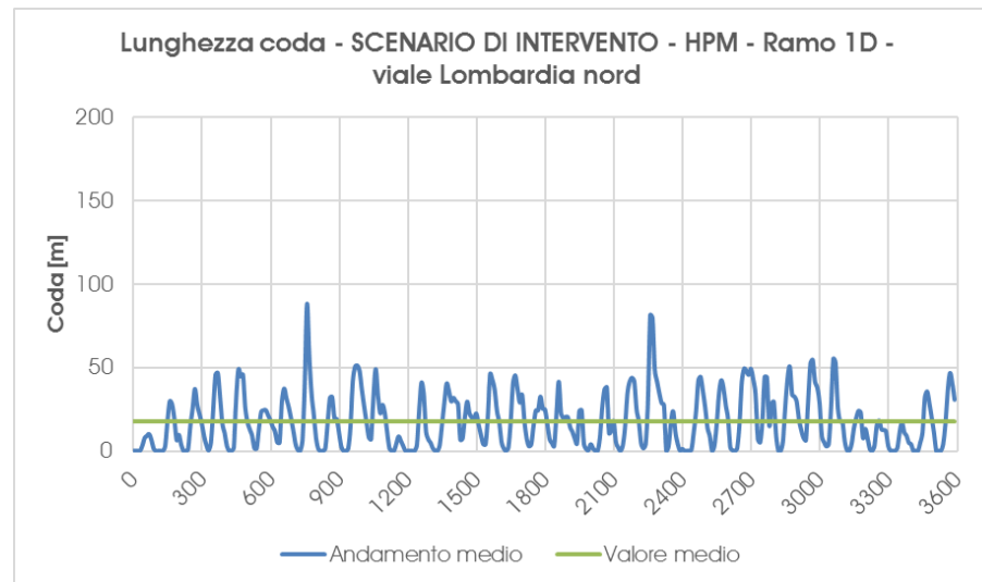
Grafico 14 – Scenario di Intervento – Accodamento medio – ramo 1D – Ora di punta della mattina
