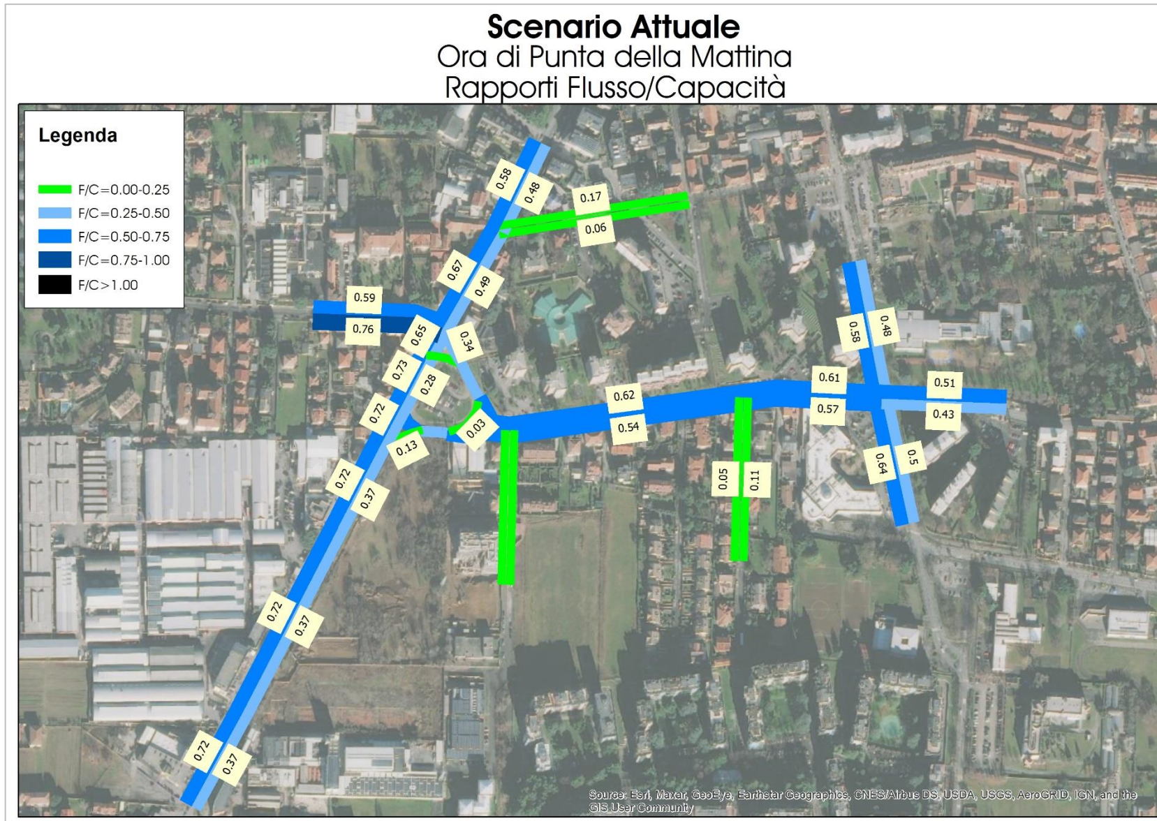
Figura 31 – Scenario Attuale – Ora di punta della mattina – Rapporti Flusso/Capacità
