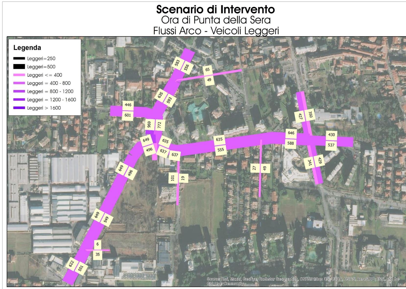
Figura 48 – Scenario di Intervento – Ora di punta della sera – Flussogramma – Veicoli Leggeri
