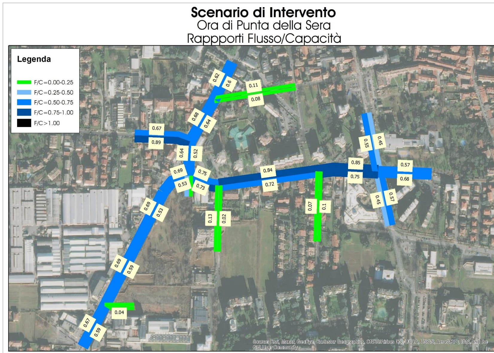
Figura 50 – Scenario di Intervento – Ora di punta della sera – Rapporti Flusso/Capacità
