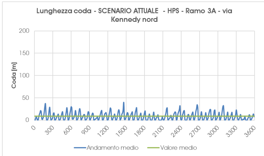
Grafico 33 – Scenario Attuale – Accodamento medio – ramo 3A – Ora di punta della sera
