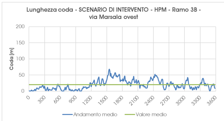
Grafico 26 – Scenario Attuale – Accodamento medio – ramo 3B – Ora di punta della mattina
