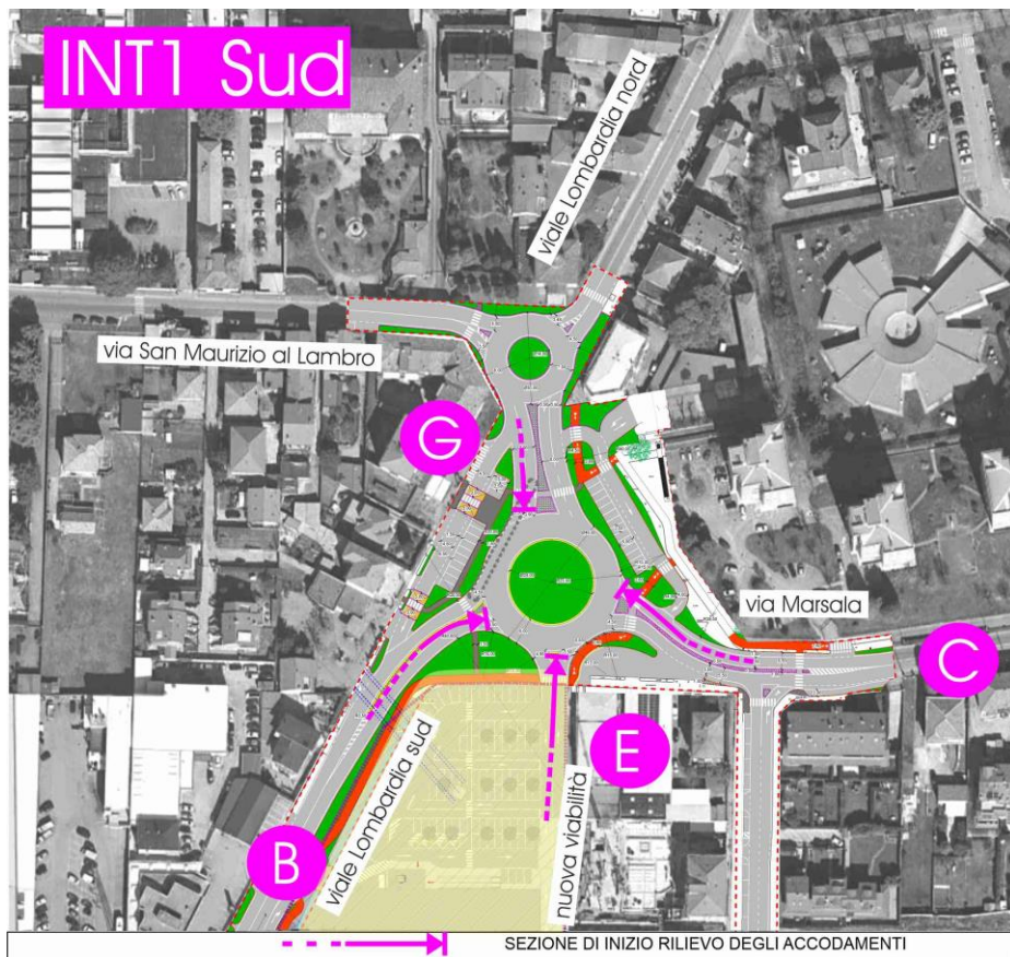
Figura 61 – Scenario di Intervento – Intersezione 1 Sud
