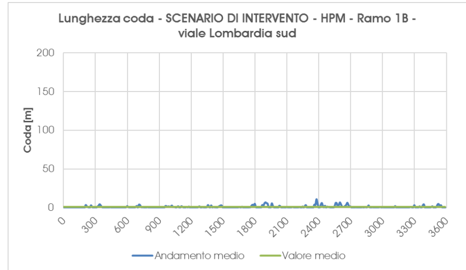
Grafico 10 – Scenario di Intervento – Accodamento medio – ramo 1B – Ora di punta della mattina
