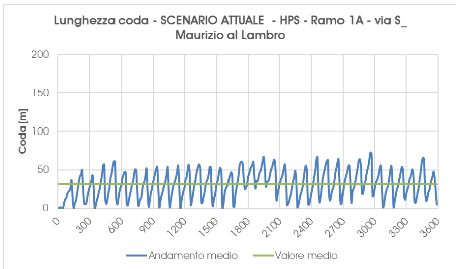
Grafico 15 – Scenario Attuale – Accodamento medio – ramo 1A – Ora di punta della sera
