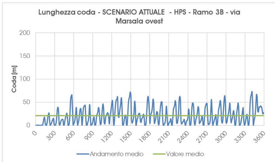
Grafico 36 – Scenario Attuale – Accodamento medio – ramo 3B – Ora di punta della sera
