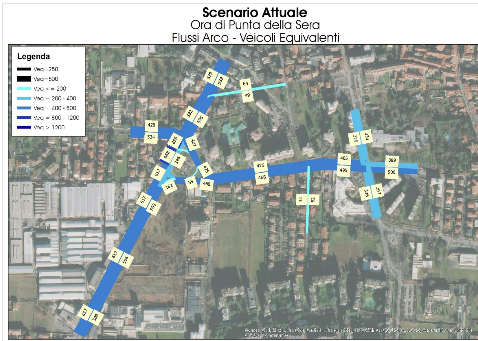
Figura 32 – Scenario Attuale – Ora di punta della sera – Flussogramma
