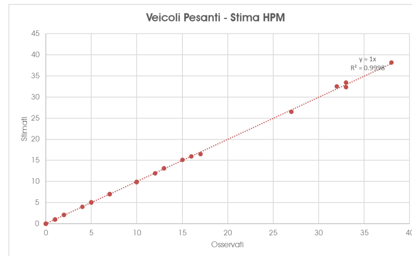
Grafico 4 – Scenario Attuale HPM – Confronto flussi osservati e flussi stimati (pesanti)
