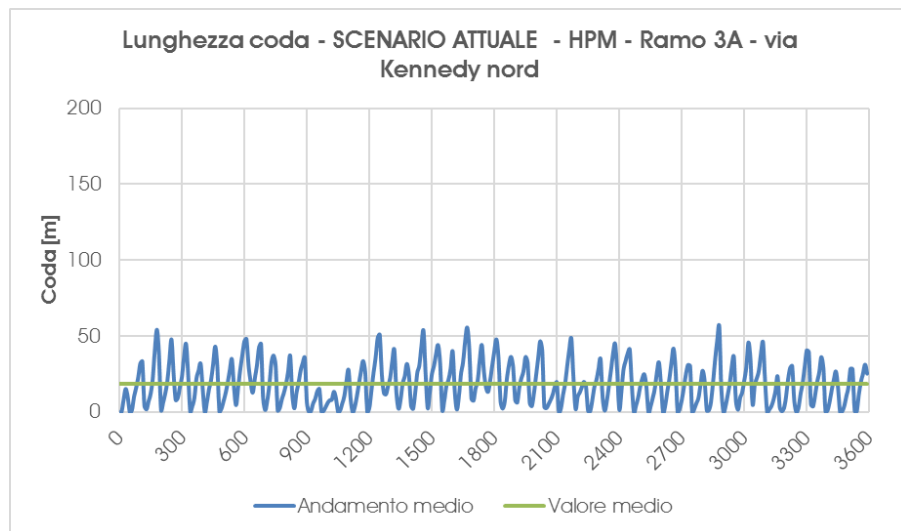
Grafico 23 – Scenario Attuale – Accodamento medio – ramo 3A – Ora di punta della mattina
