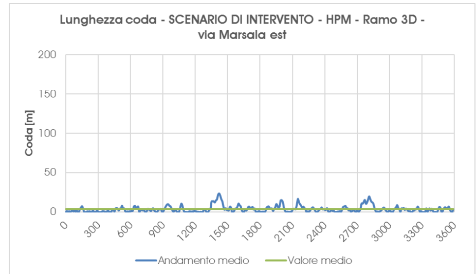
Grafico 32 – Scenario di Intervento – Accodamento medio – ramo 3D – Ora di punta della mattina
