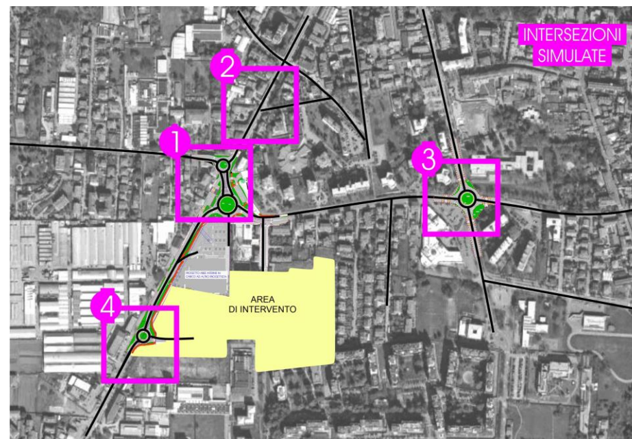
Figura 58 – Scenario di Intervento – Intersezioni analizzate con il modello di simulazione microscopica
