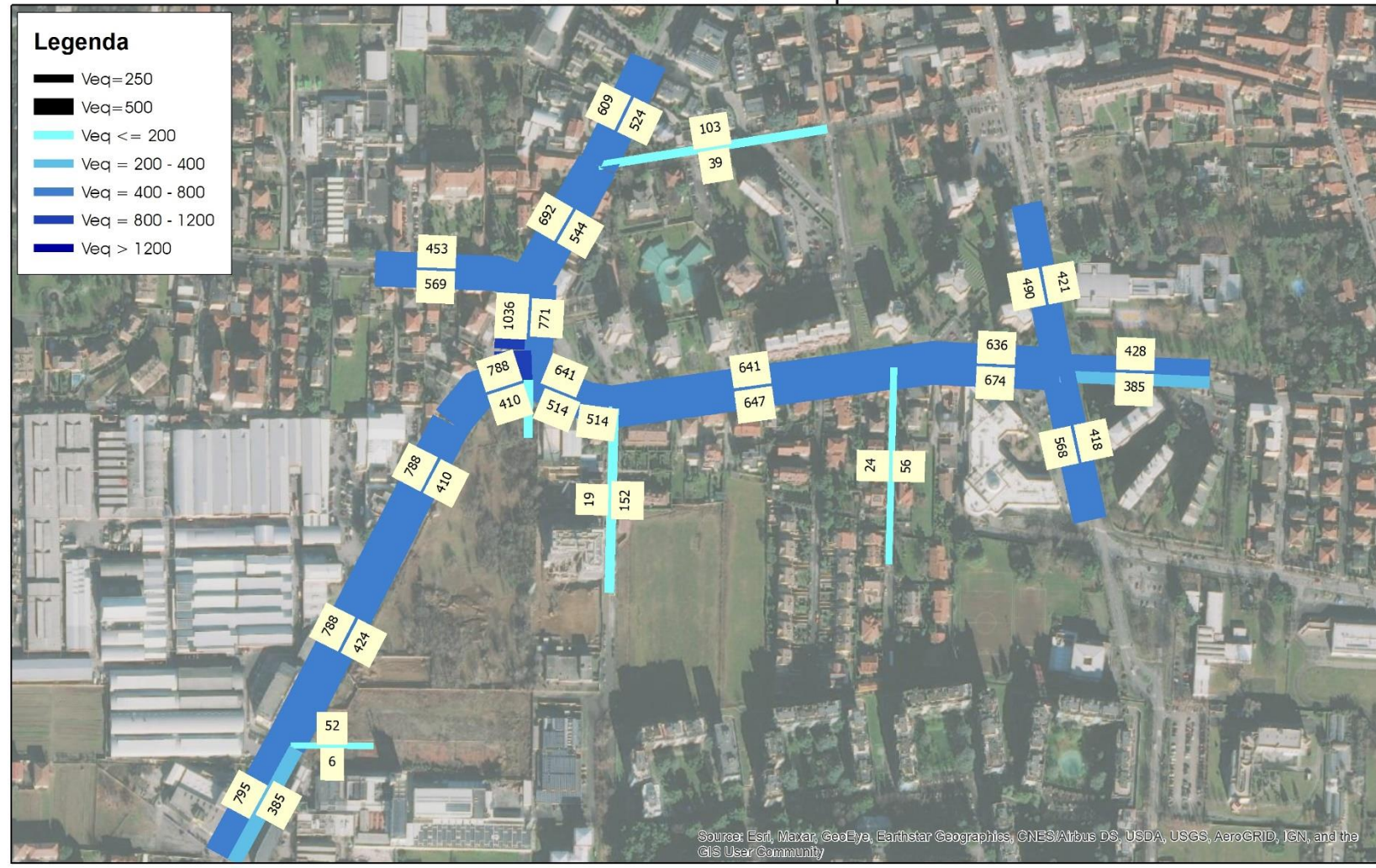
Figura 42 – Scenario di Intervento – Ora di punta della mattina – Flussogramma
