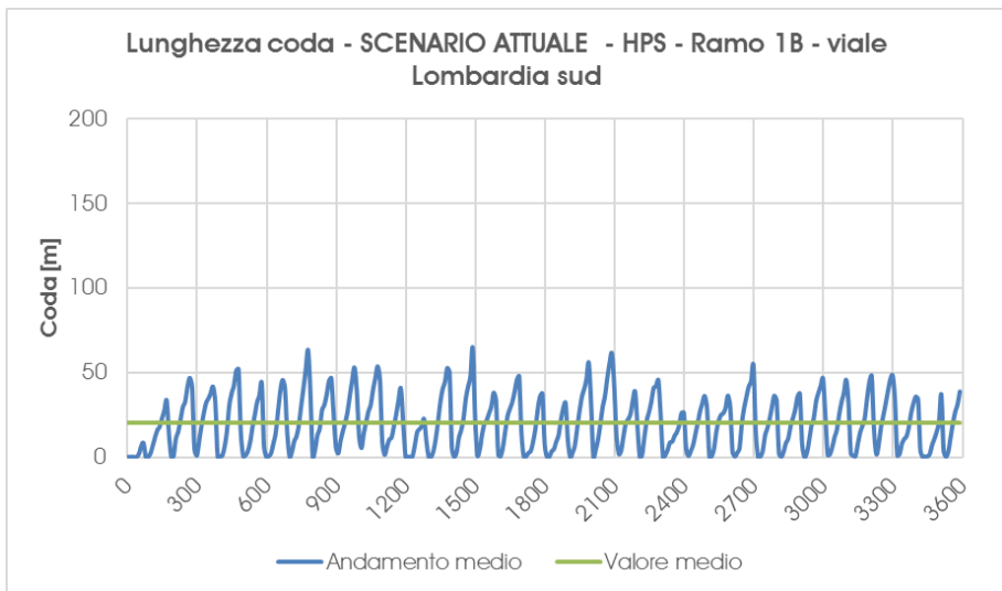
Grafico 16 – Scenario Attuale – Accodamento medio – ramo 1B – Ora di punta della sera
