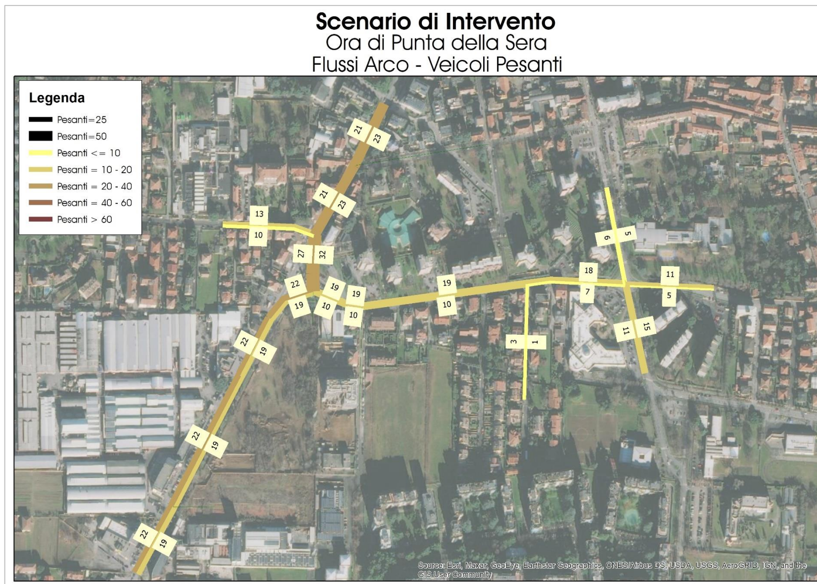
Figura 49 – Scenario di Intervento – Ora di punta della sera – Flussogramma – Veicoli Pesanti
