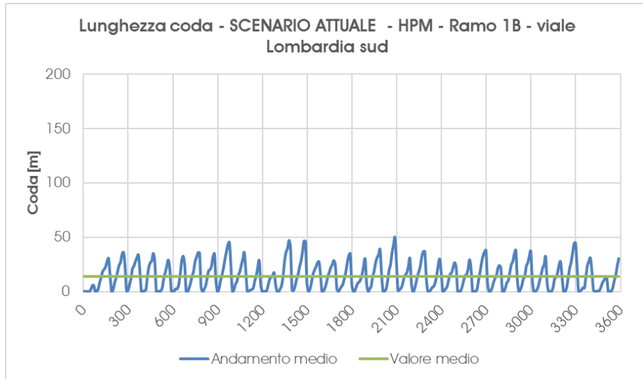
Grafico 8 – Scenario Attuale – Accodamento medio – ramo 1B – Ora di punta della mattina
