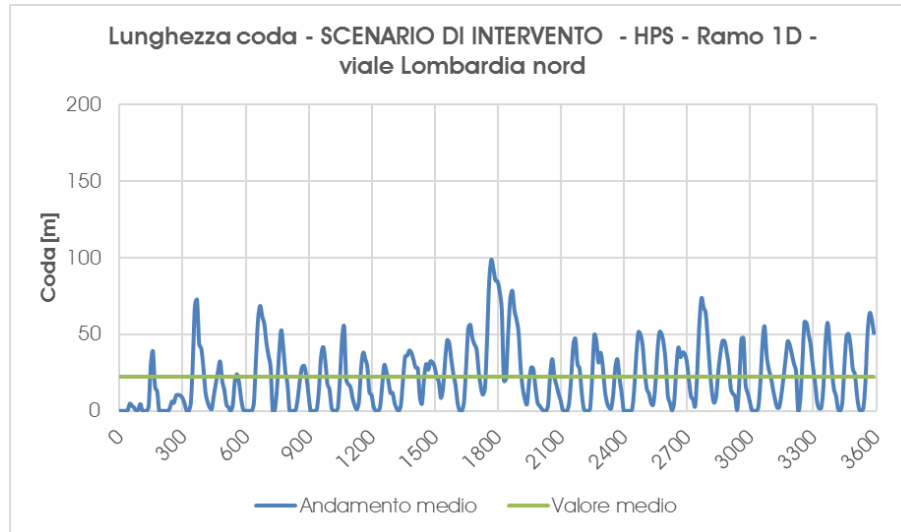
Grafico 22 – Scenario di Intervento – Accodamento medio – ramo 1D – Ora di punta della sera
