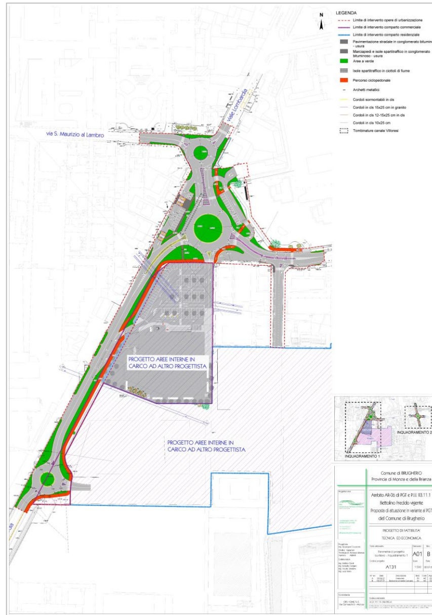
Figura 37 – Scenario di Intervento – Opere Viabilistiche Proposta di attuazione in variante al PGT Ambito AR-06 di PGT e P.I. B3.11.1 Bettolino Freddo vigente – Inquadramento 1
