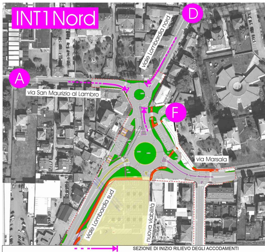
Figura 60 – Scenario di Intervento – Intersezione 1 Nord
