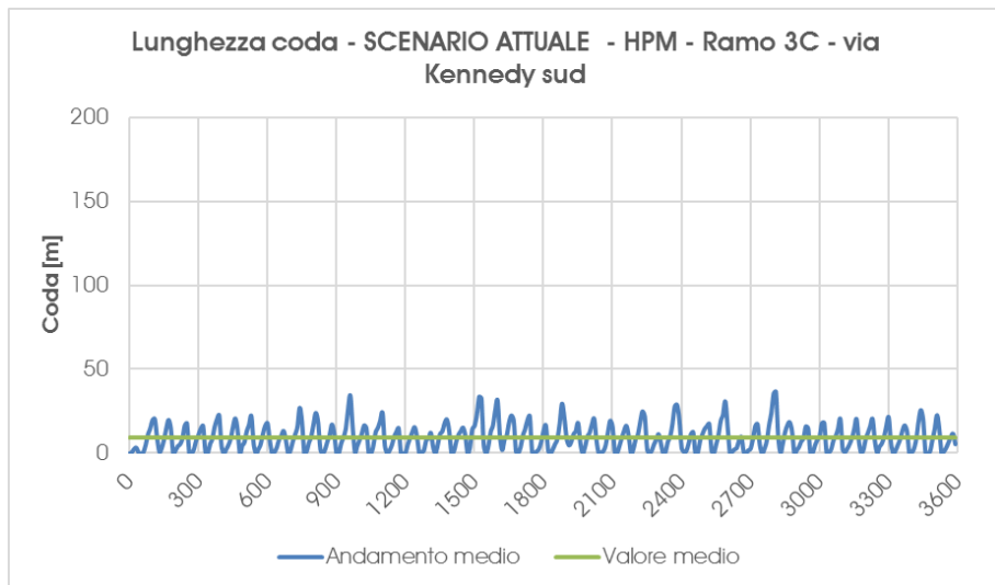
Grafico 27 – Scenario Attuale – Accodamento medio – ramo 3C – Ora di punta della mattina
