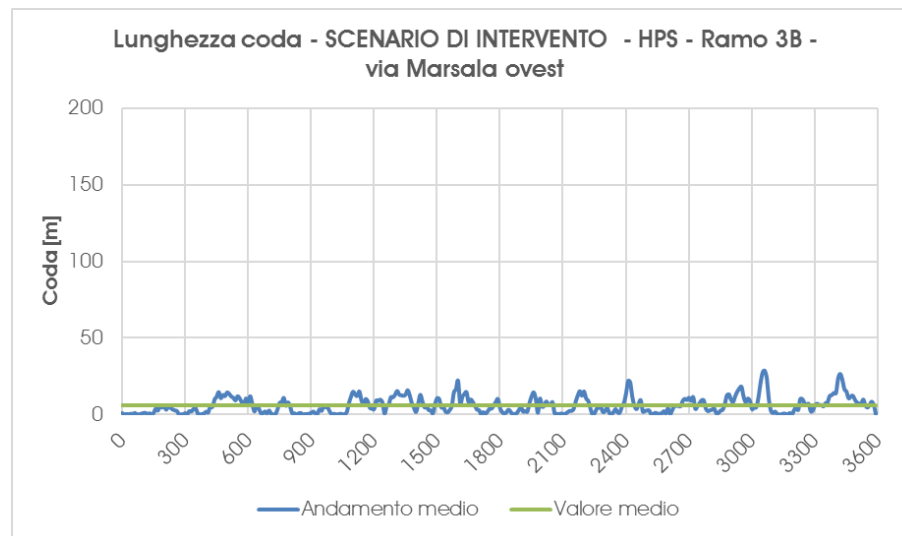
Grafico 38 – Scenario di Intervento – Accodamento medio – ramo 3B – Ora di punta della sera
