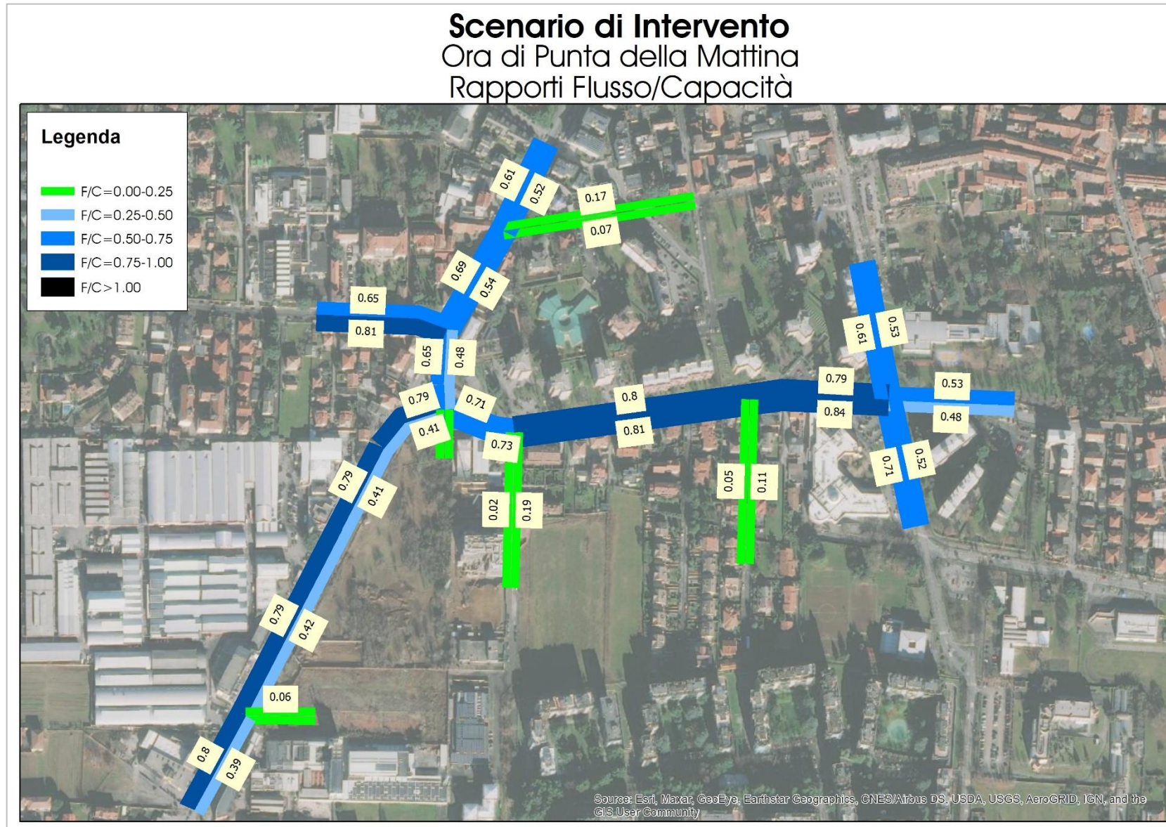
Figura 45 – Scenario di Intervento – Ora di punta della mattina – Rapporti Flusso/Capacità
