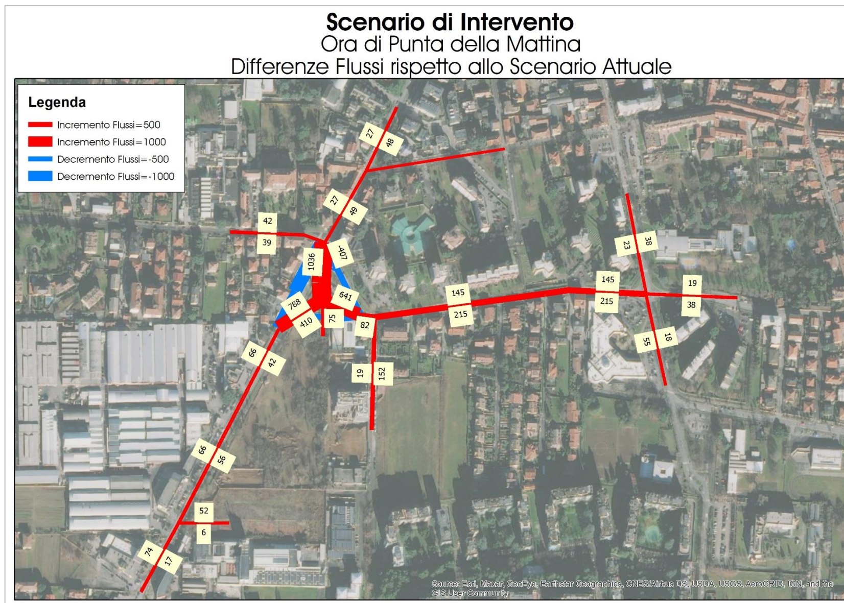
Figura 46 – Scenario di Intervento – Ora di punta della mattina – Differenze Flussi rispetto allo Scenario Attuale
