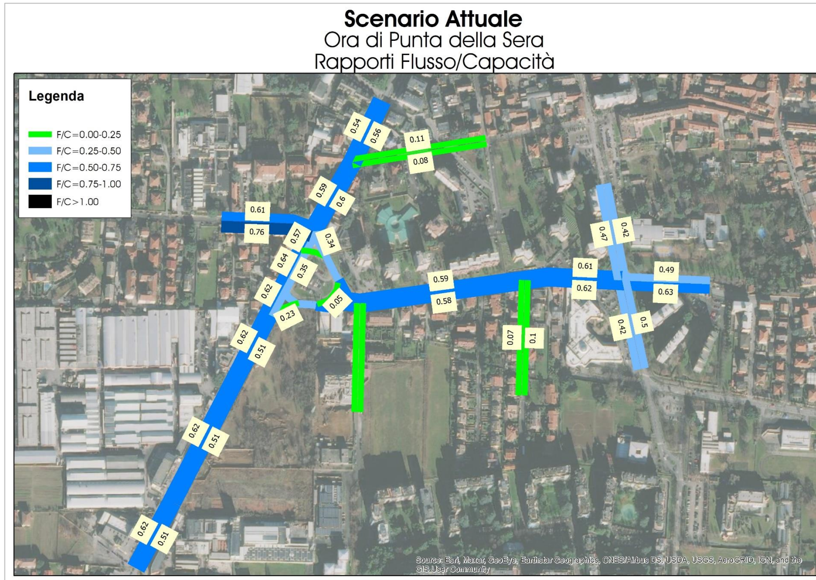
Figura 35 – Scenario Attuale – Ora di punta della sera – Rapporti Flusso/Capacità
