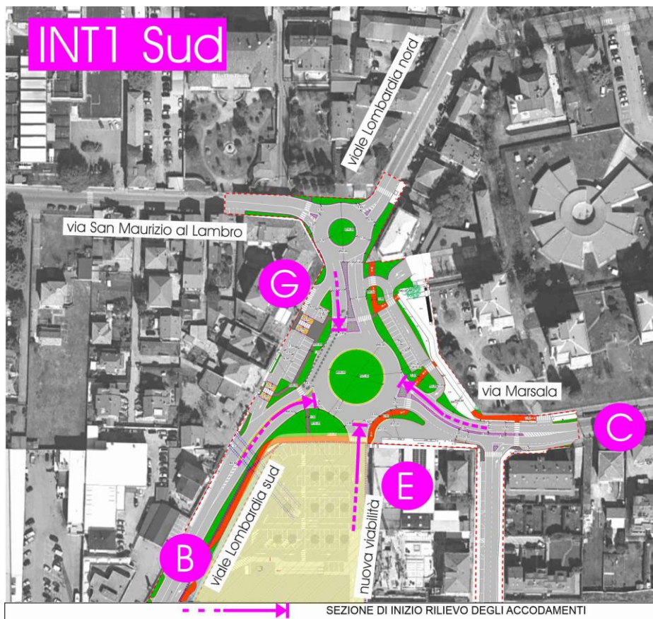
Figura 63 – Scenario di Intervento – Intersezione 1 Sud
