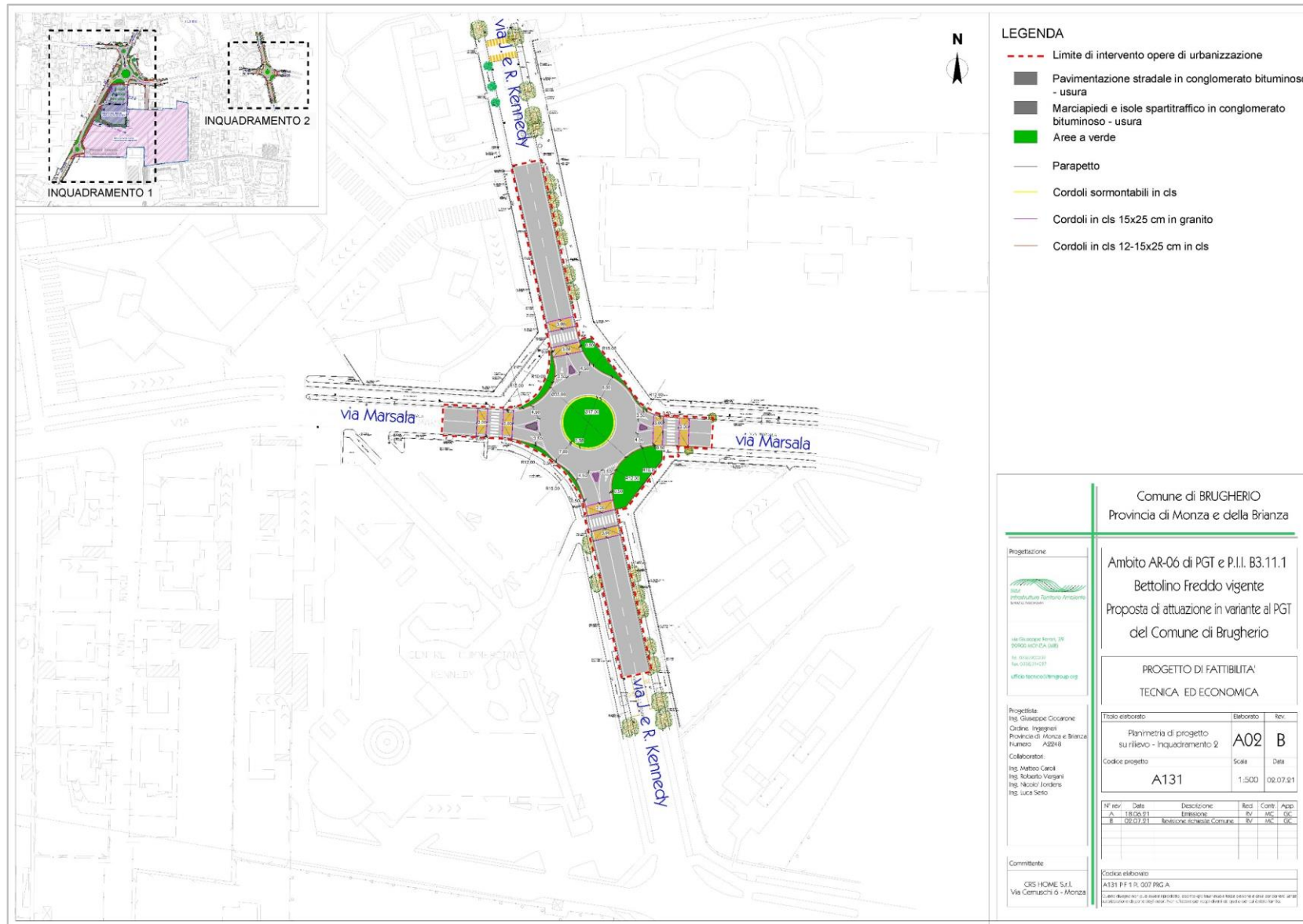
Figura 38 – Scenario di Intervento – Opere viabilistiche Proposta di Attuazione in variante al PGT Ambito AR-06 di PGT e PII B3.11.1 Bettolino Freddo vigente – Inquadramento 2
